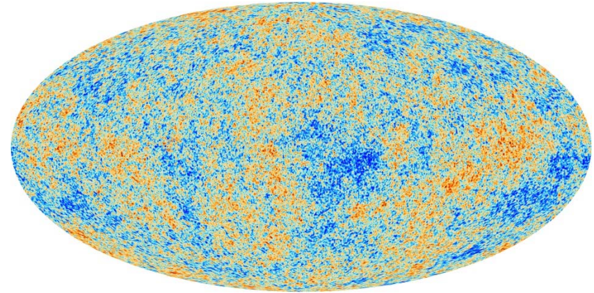
宇宙背景放射 (Planck HPより)
